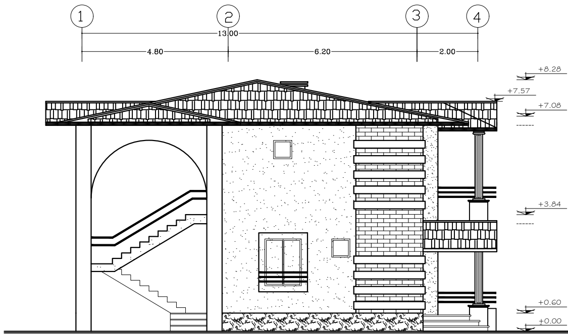
نمای جانبی
