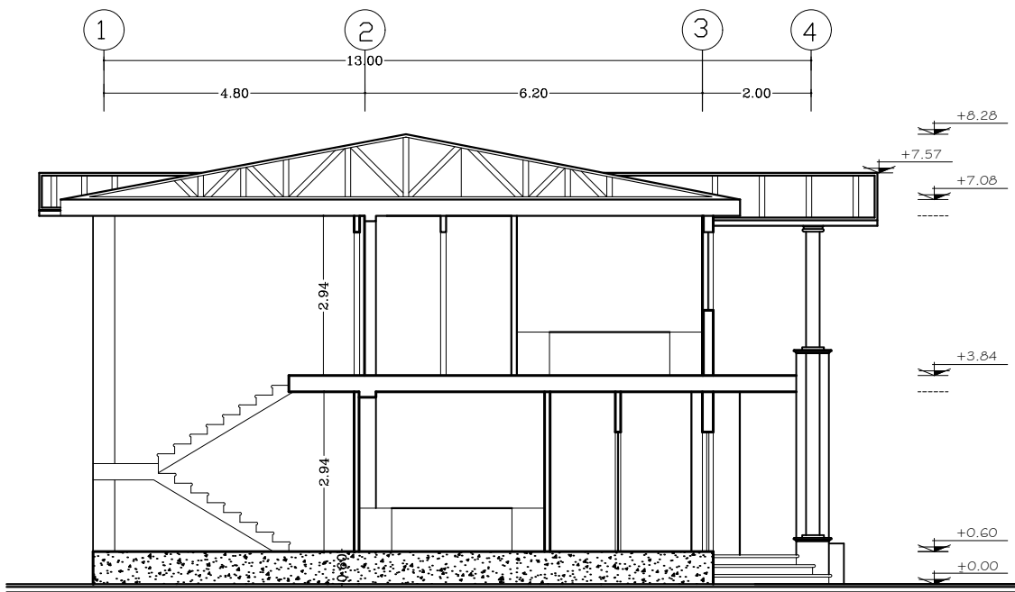
برش
