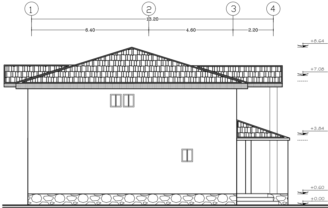
نمای جانبی
