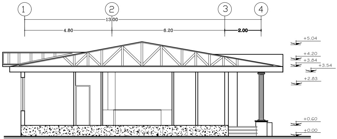
نمای جانبی
