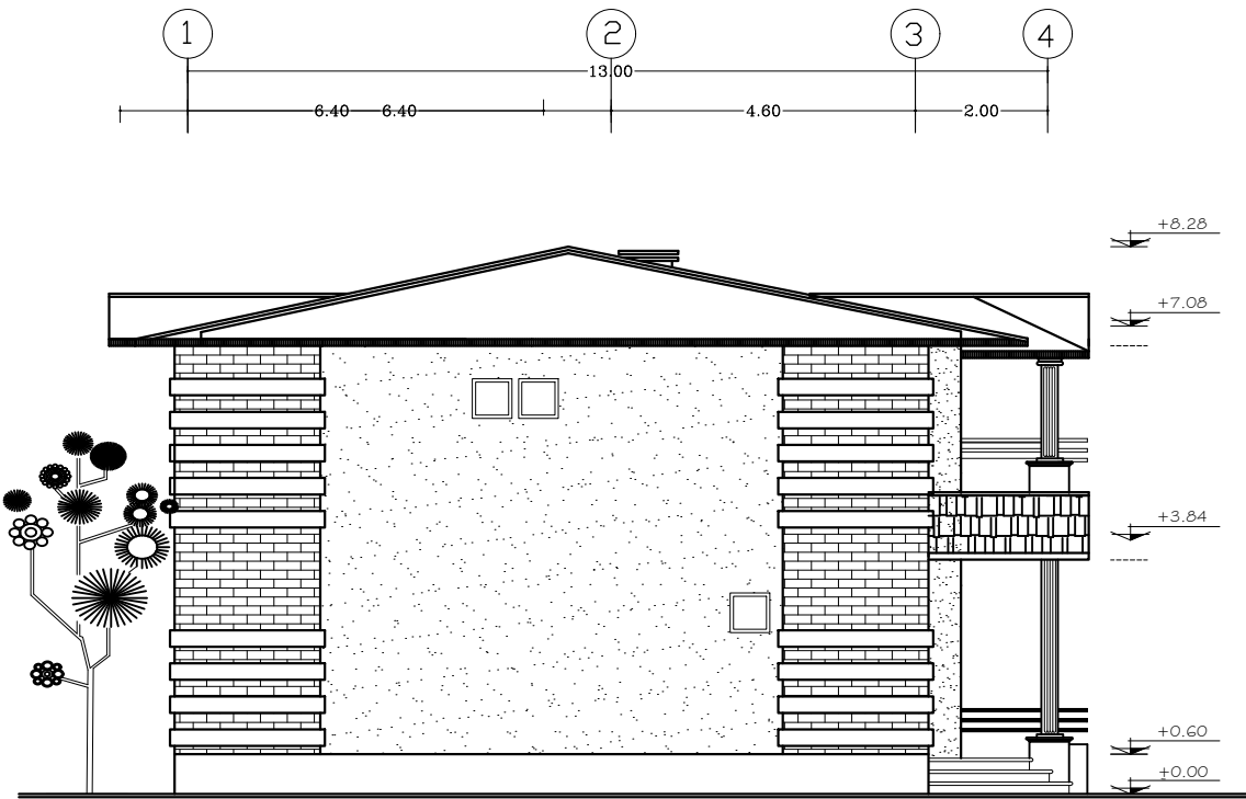
نمای جانبی
