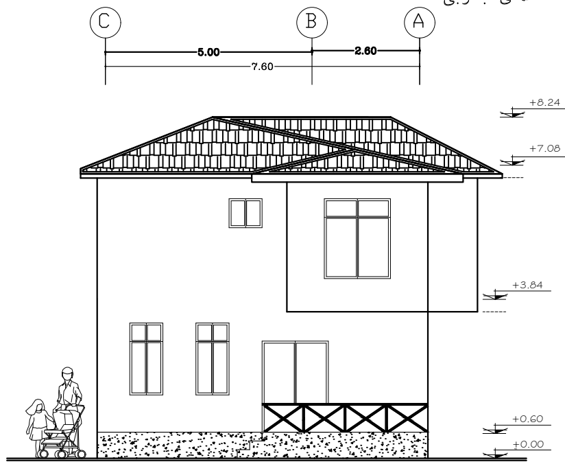
نمای شمالی
